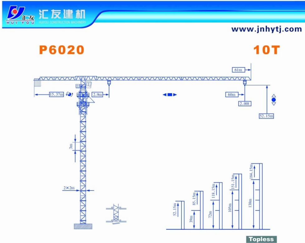
起重量载荷表 Load Capacity
