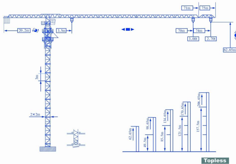
起重载荷表 Load Capacity
