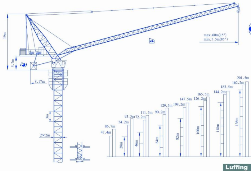
起重量载荷表 Load Capacity
