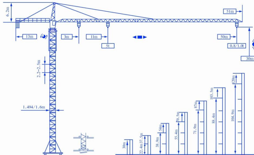
起重量载荷表 Load Capacity
